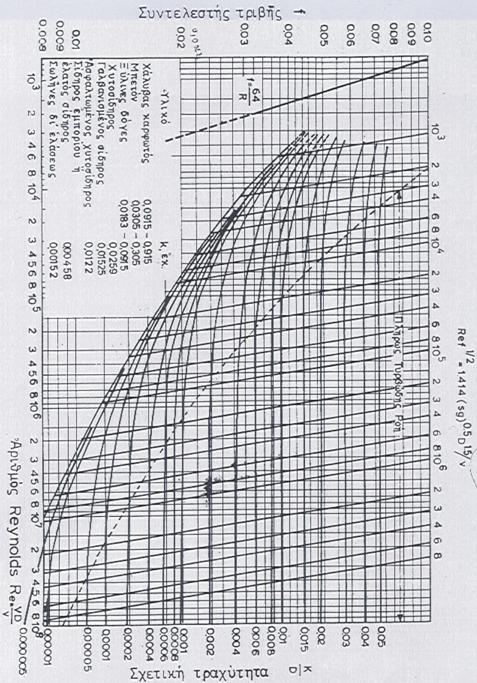
Σχ. Α Διάγραμμα Moody (Darcy-Hartmann 1966)
